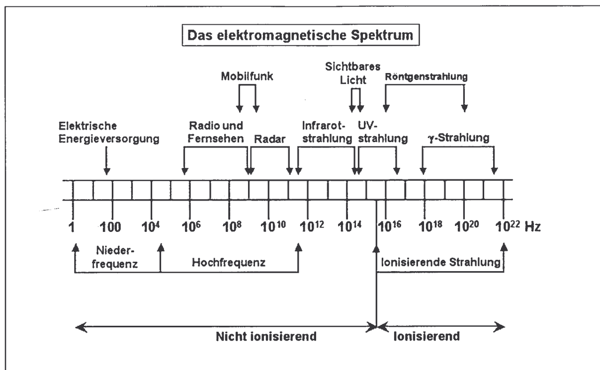
ABBILDUNG 1: Das elektromagnetische Spektrum (modifiziert nach Repacholi, 1996). Das elektromagnetische Spektrum wird in Frequenzbereiche mit sehr unterschiedlichen Eigenschaften und biologischen Wirkungen unterteilt. Zu den statischen Feldern (0 Hertz) gehört z. B. das natürliche Erdmagnetfeld. Künstlich erzeugte statische Magnetfelder werden u. a. zur Kernspintomographie verwendet. Der Bereich der niederfrequenten Felder enthält u. a. elektrische oder magnetische Felder im extrem niedrigen Frequenzbereich von > 0 bis 300 Hertz. In diesem Frequenzbereich liegt z. B. der Wechselstrom mit 50 oder 60 Hertz. Hochfrequente elektromagnetische Felder (im Englischen auch als „Radiofrequency [RF] fields“ bezeichnet) haben Frequenzen zwischen 30 000 Hertz und 300 Giga-Hertz. Wie bei statischen oder niederfrequenten Feldern gilt die Energie dieser Felder i. G. zu UV-Licht und ionisierender Strahlung als zu schwach, um Moleküle zu ionisieren oder chemische Bindungen zu brechen und damit direkte DNS-Schädigungen hervorzurufen. RF-Felder werden für alle Arten von Informationsübertragung, also Radio (AM, FM), Fernsehen, Mobilfunk und Radar verwendet. Erst oberhalb dieses Hochfrequenzbereiches spricht man von Strahlung. Immer noch im nicht-ionisierenden Bereich (von \sim 10^{12} – 10^{17} Hertz) liegt die optische Strahlung, zu der Infrarot, sichtbares Licht und UV-Strahlung gehören. Im Frequenzbereich von > 10^{15} – 10^{22} liegt die ionisierende Strahlung (Röntgen- und Gamma-Strahlung).
